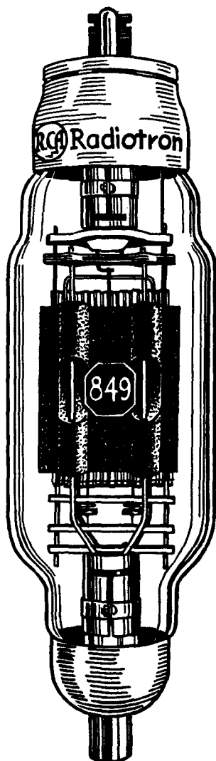
RCA-849
