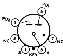
4R Type 0Z4
