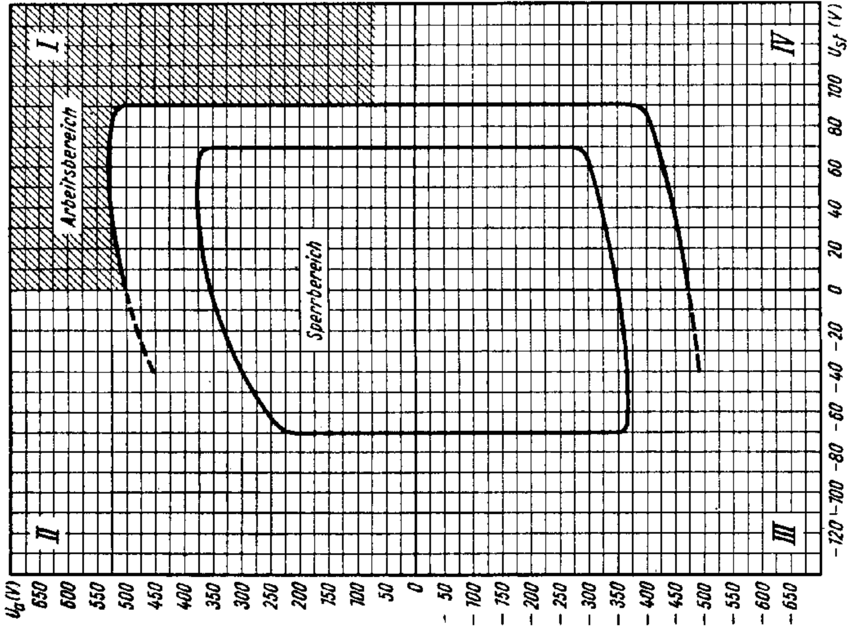
Zünddiagramm
